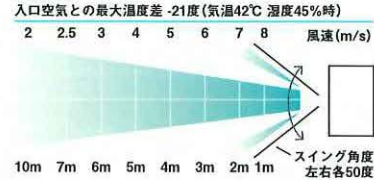
風速図
