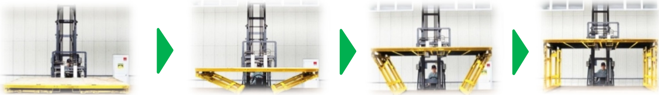
【組み立て】
